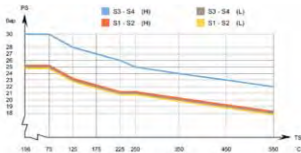
Диаграмма "давление-температура" для модели AlfaNova 27 (соответствует нормативам PED)
