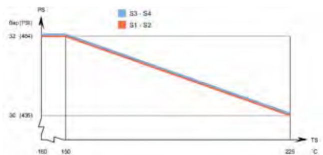
Диаграмма "давление–температура" для модели СВН16 (соответствует нормативам PED)
