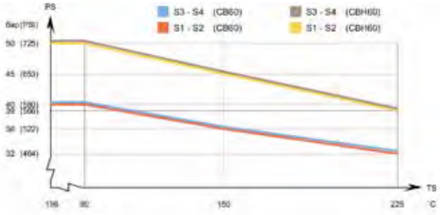
Диаграмма “давление–температура” для модели CB60/CBH60 (соответствует нормативам PED)
