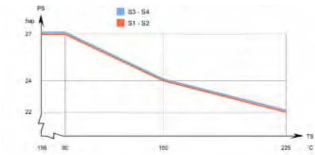
Диаграмма "давление-температура" для модели СВН110 (соответствует нормативам PED)
