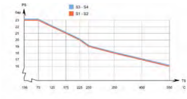
Диаграмма “давление–температура” для модели AlfaNova 14 (соответствует нормативам PED)
