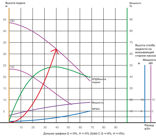
Характеристики насоса (50 Гц)
