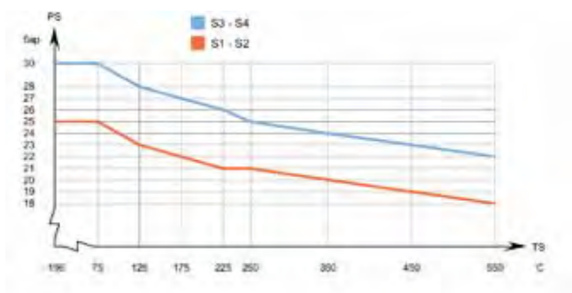
Диаграмма “давление–температура” для модели AlfaNova 52* (соответствует нормативам PED)
