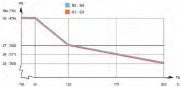
Диаграмма “давление–температура” для модели СВ200 (соответствует нормативам PED)
