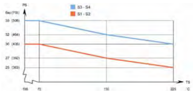
Диаграмма “давление–температура” для модели СВ400 (соответствует нормативам PED)
