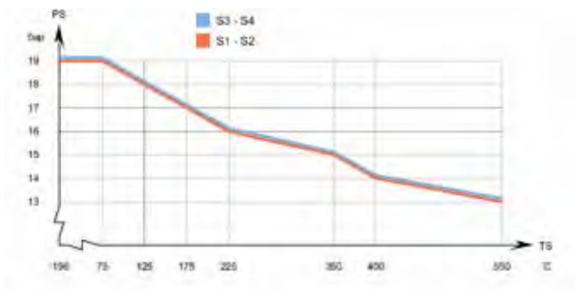
Диаграмма "давление-температура" для модели AlfaNova 400* (соответствует нормативам PED)
